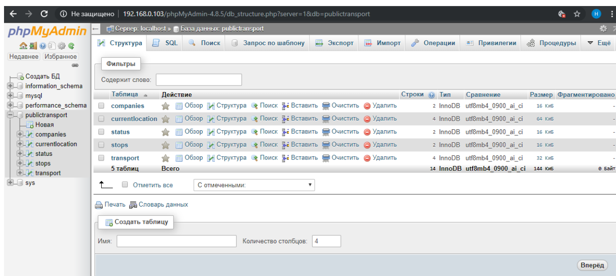
Рисунок 4.2.1 – интерфейс phpMyAdmin
