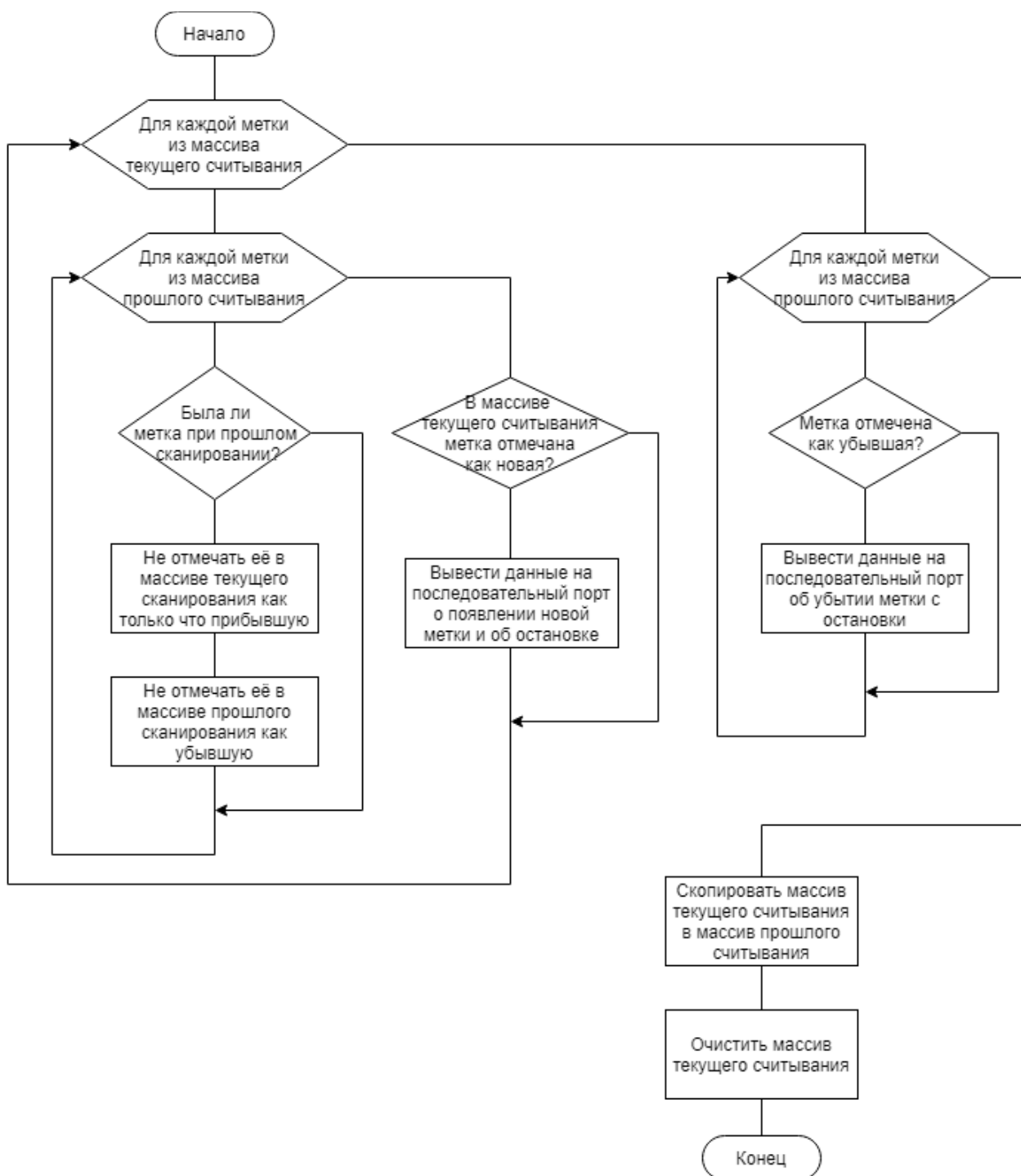
Рисунок 3.2.3 – алгоритм обработчика прерывания
