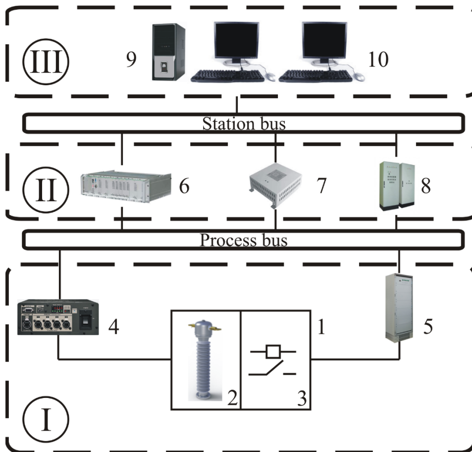
Рисунок 1 – АЦКТН в структуре ЦПС (добавить 12, 13 из ИБ)
