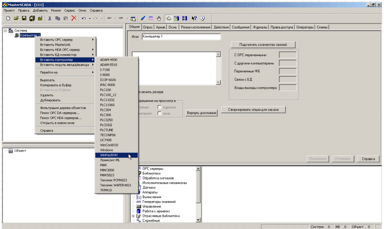
Рисунок 4 — Выбор контроллера средствами MasterSCADA
