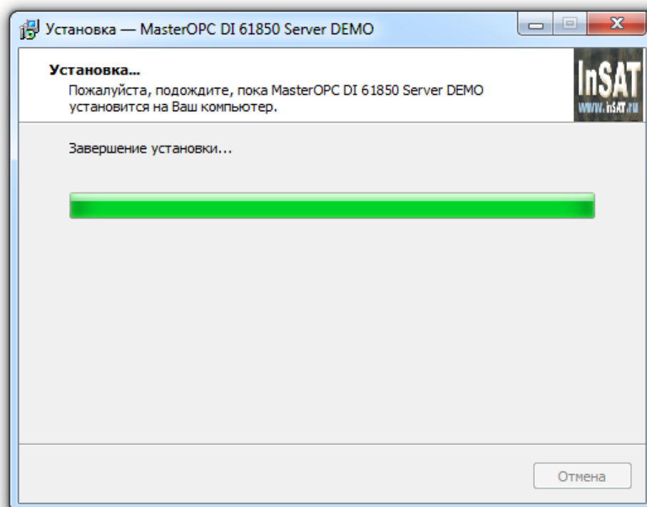
Рисунок 35 — Окно установки
