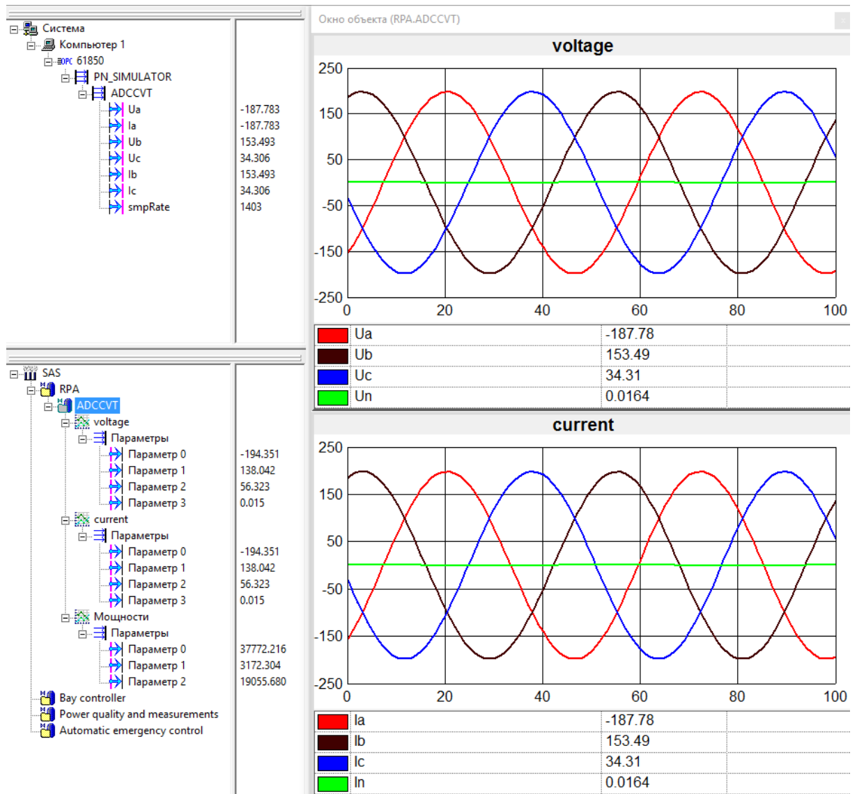
Рисунок 47 — Кривые напряжения и тока для состояния «Нормальные условия»
