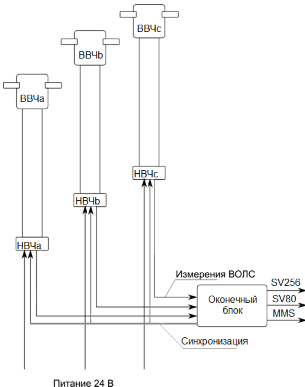
Рисунок 2 – Функциональная схема измерительной системы на основе АЦКТН
