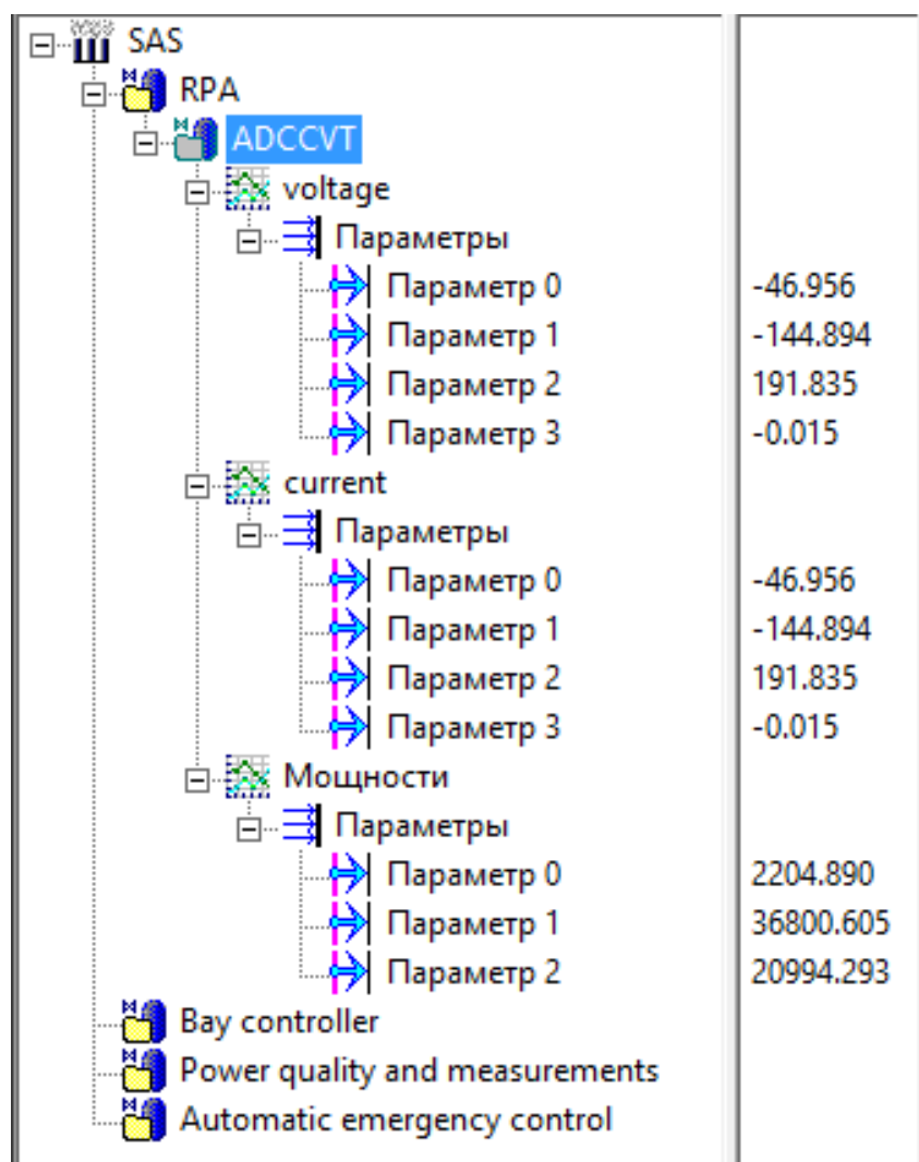
Рисунок 41 – Дерево объектов
