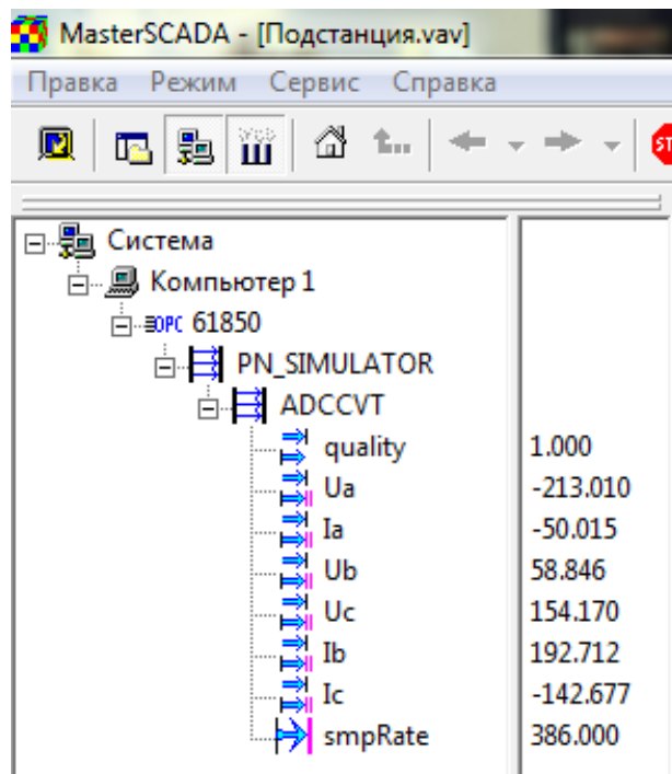
Рисунок 17 — Дерево системы
