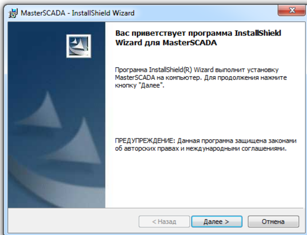
Рисунок 24 — Окно приветствия
