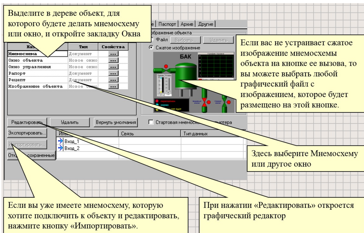
Рисунок 6 — Создание мнемосхем
