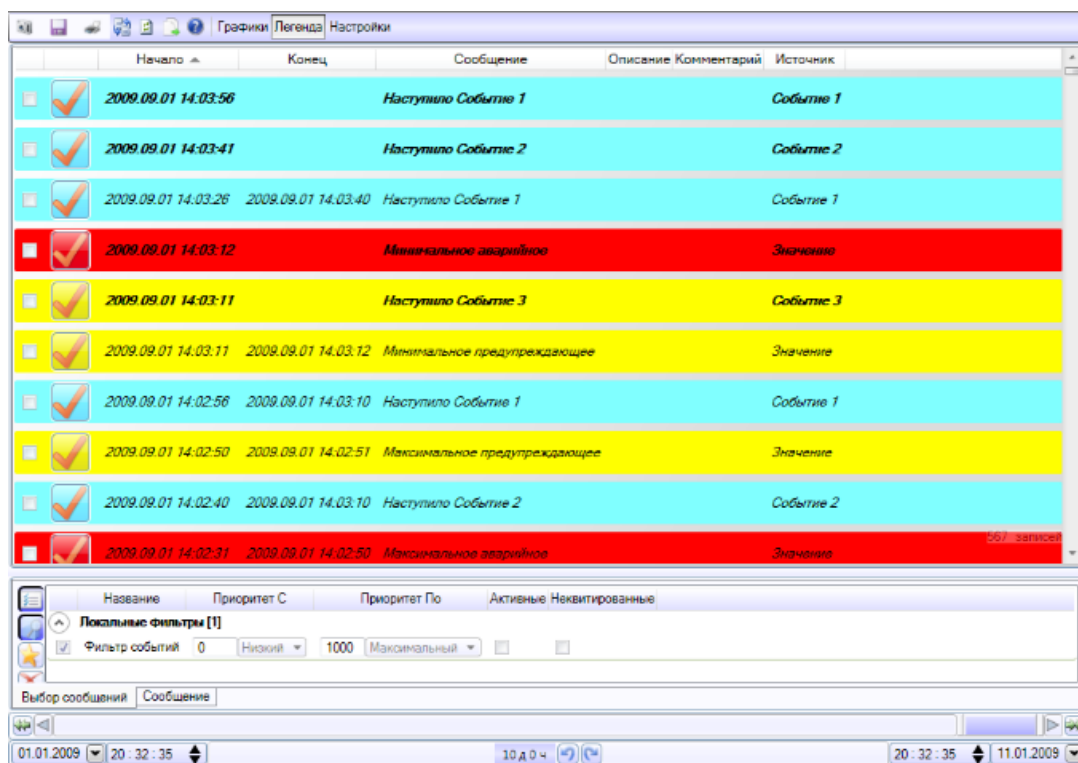
Рисунок 8 — Журнал сообщений
