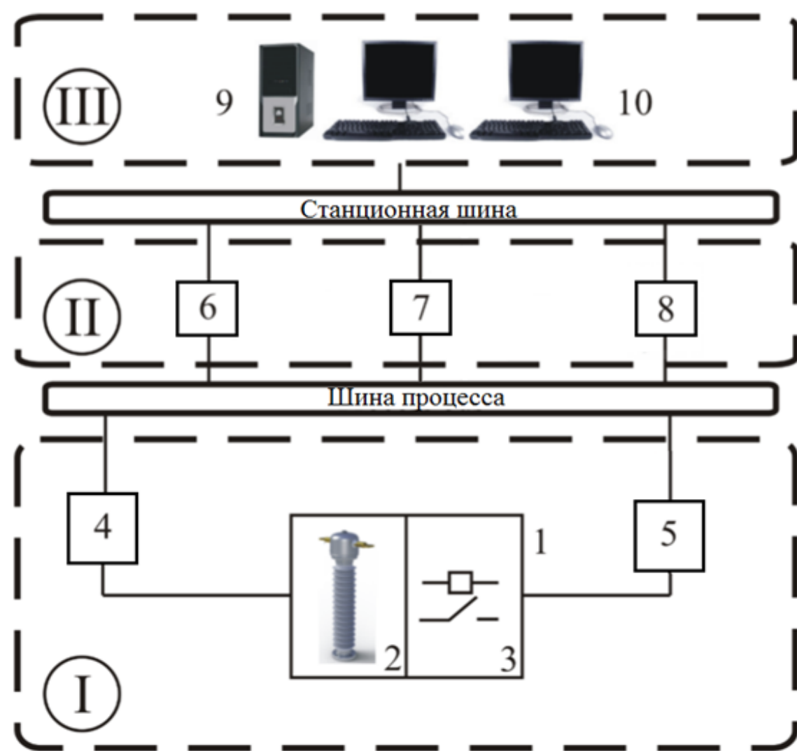
Рисунок 40 — Топология сети АЦКТТН
