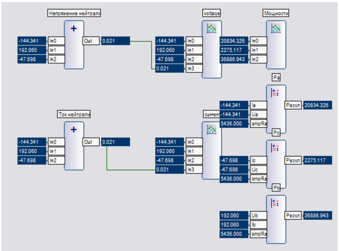
Рисунок 42 — Уровень процесса
