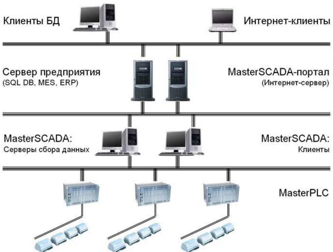
Рисунок 15 — Сетевая структура MasterSCADA
